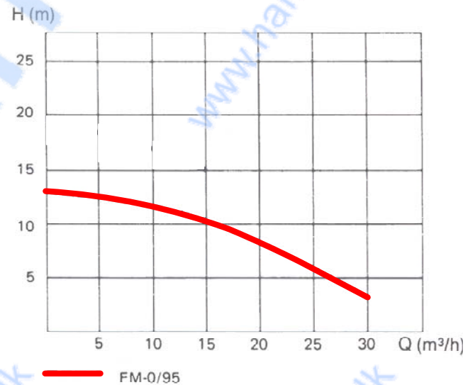
Fig. 2. Kapacitetsdiagram.
